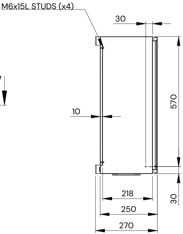
SECTION AV-AV
