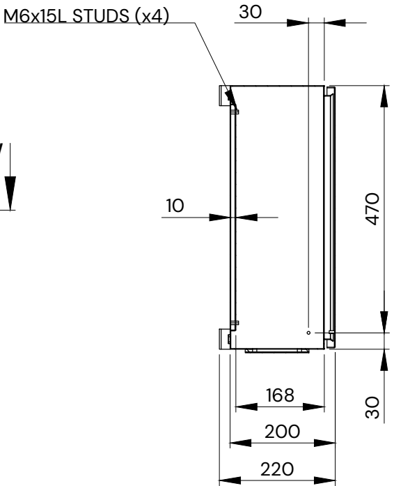
SECTION AV-AV
