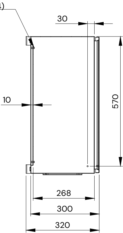
SECTION AV-AV
